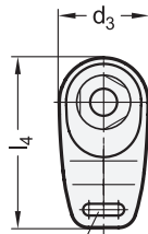
Halka için oluklu delik (Bilye zincir)
